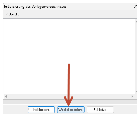
Abbildung 2: Neue Reparaturfunktion
