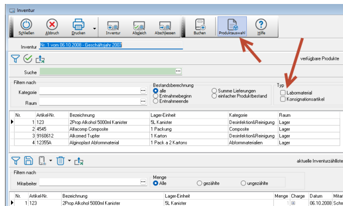
Abbildung 4: Filterung nach Labor
