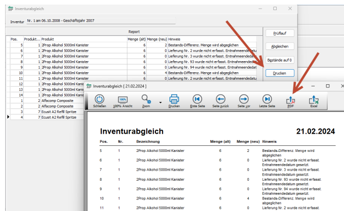
Abbildung 5: Abschlussreport
