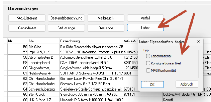
Abbildung 3: Laboreigenschaften ändern
