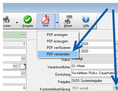
Abbildung 4: PDF-Konformitätserklärung versenden
