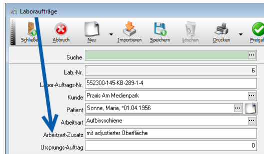
Abbildung 1: Neu: Arbeitsart-Zusatz
