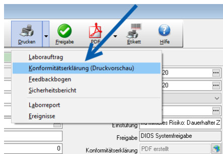
Abbildung 5: Eingeschränkte Druckvorschau
